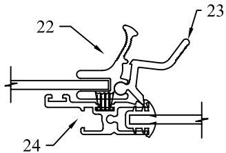
SECTION D-D Optional Center Latch
