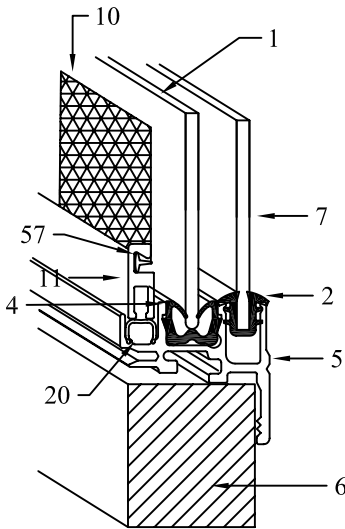
SECTION D-D Optional Center Latch
